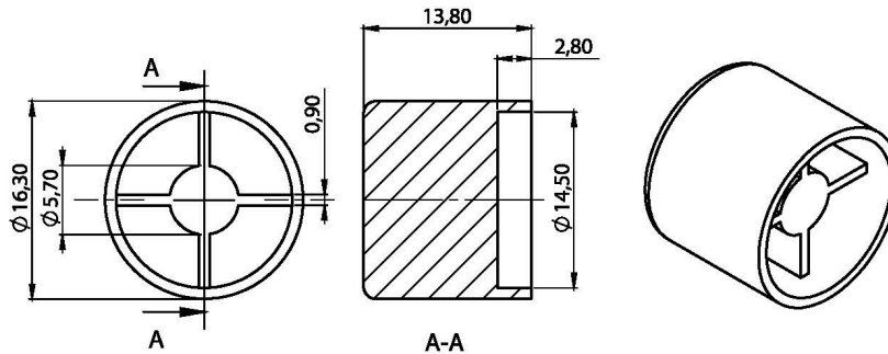
KNOB
